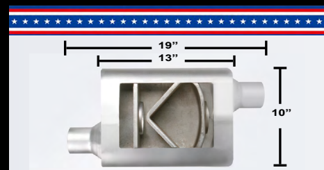
4"x10"x13" OFFSET/OFFSET
