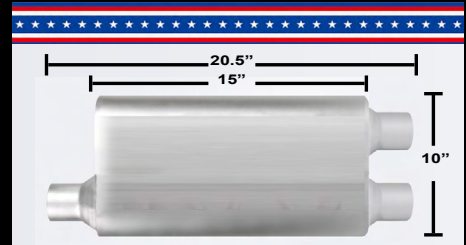
4"x10"x15" CAMARO
